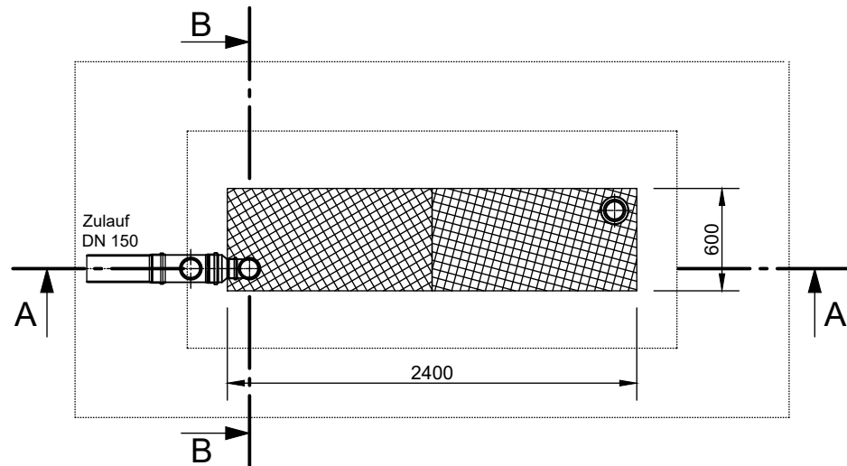
Grundriss
