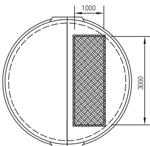
Detail: Abdeckung aus nicht rostendem Stahl
