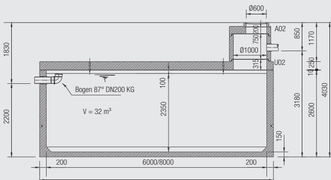
Oval-Schachtbauwerk
