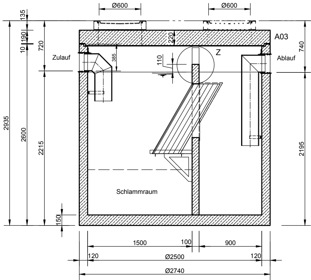
Schnitt A-A
