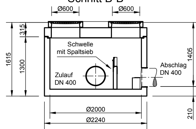
Schnitt B-B
