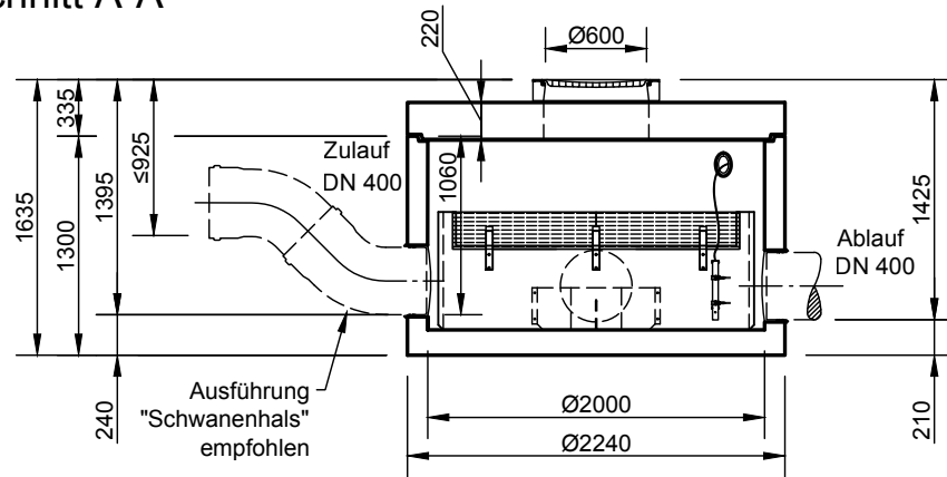
Schnitt A-A
